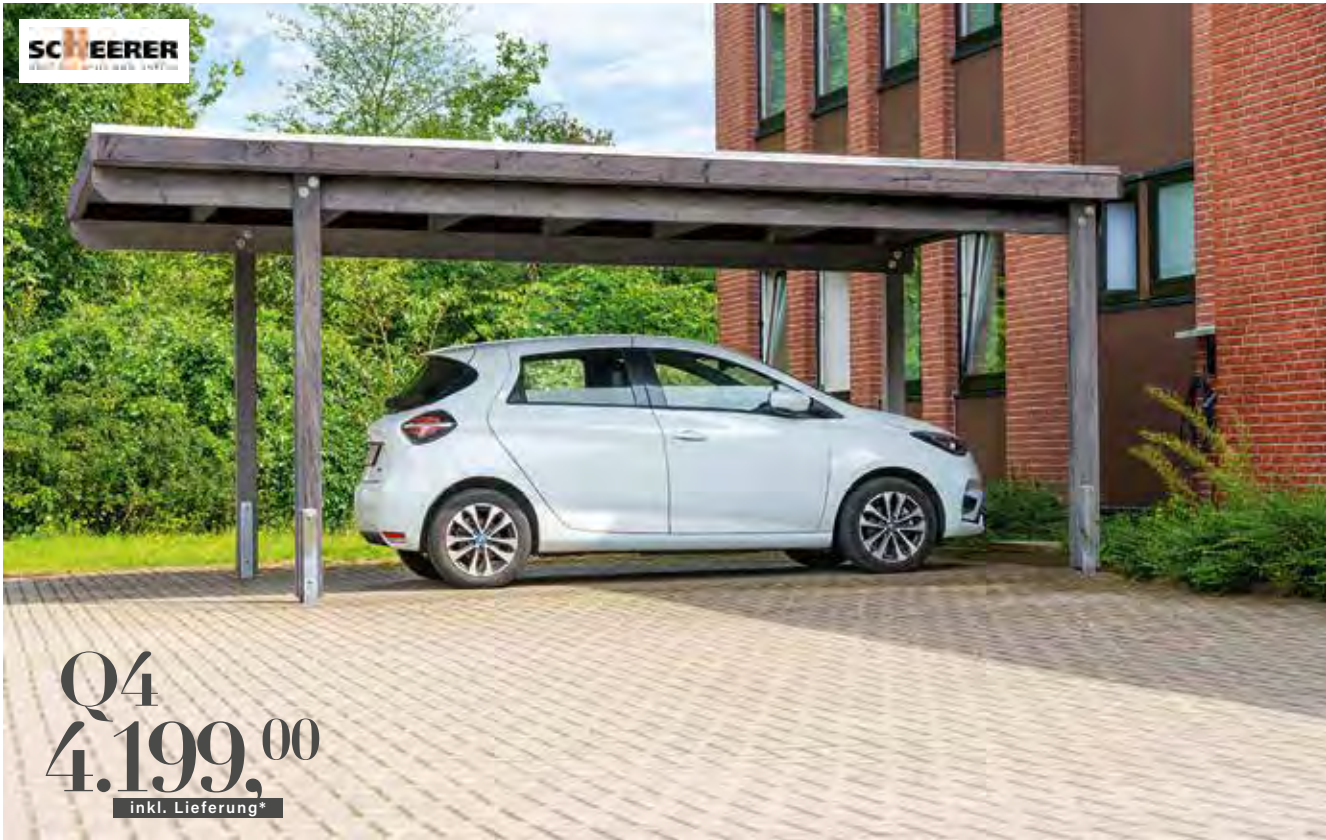
Carport Q4 aus kesseldruckimprägniertem Kiefern-/Fichtenleimholz, grau, Dacheindeckung Alu-Trapezplatten mit Antitropfschutz, Fallrohr in Anthrazit, 4 Leimholzpfeosten 14 x 14 cm, H-Bodenanker zum Einbetonieren separat erhältlich, Einfahrtshöhe 220 cm, Schneelast 150 kg/m², 400 x 600 cm, Art.-Nr. 3691321 4.199,00
