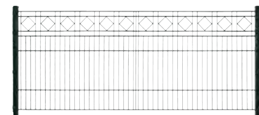
Dekormattenzaun mit Karo-Ornament B x H 246,8 x 101 cm, Art.-Nr. 1293718
