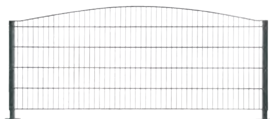
Dekormattenzaun mit Oberbogen B x H 246,8 x 103 cm, Art.-Nr. 1293720
